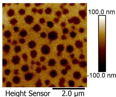
AFM-Höhenbilder einer reinen PVDF-TrFE Schicht (oben) und einer PVDF-TrFE Schicht mit zusätzlichem dünnem Polymerfilm auf der Oberfläche (unten) (Substrat: Silizium-Wafer)
